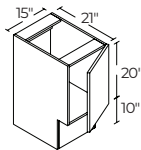
15" | V15ADA
