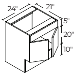
24" | VS24ADA
