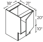
18" | V18ADA
