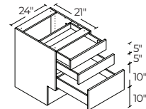
24" | V3D24ADA
