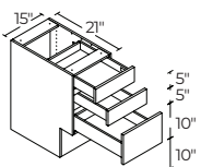
15" | V3D15ADA
