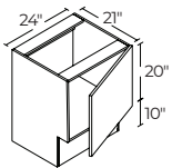
24" | V24ADA
