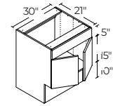
30" | VS30ADA
