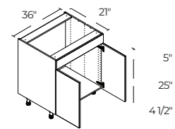
36" | VS36
