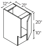
12" | V12ADA
