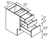
12" | V3D12ADA
