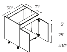
30" | VS30
